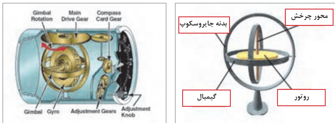
شکل ۴- ژيروسکوپ و قسمت‌های آن
