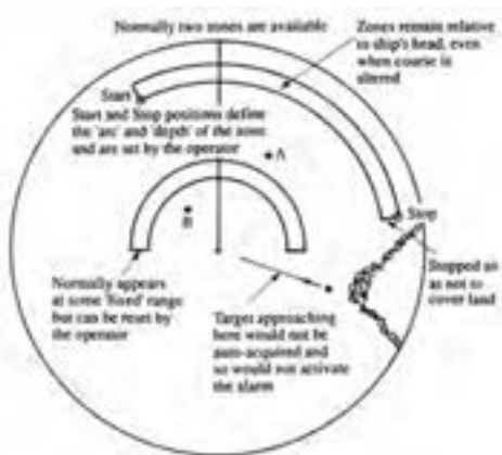
شکل ۲۴- نحوه نمایش مناطق حفاظتی (Guard zones) در صفحه نمایشگر ARPA
